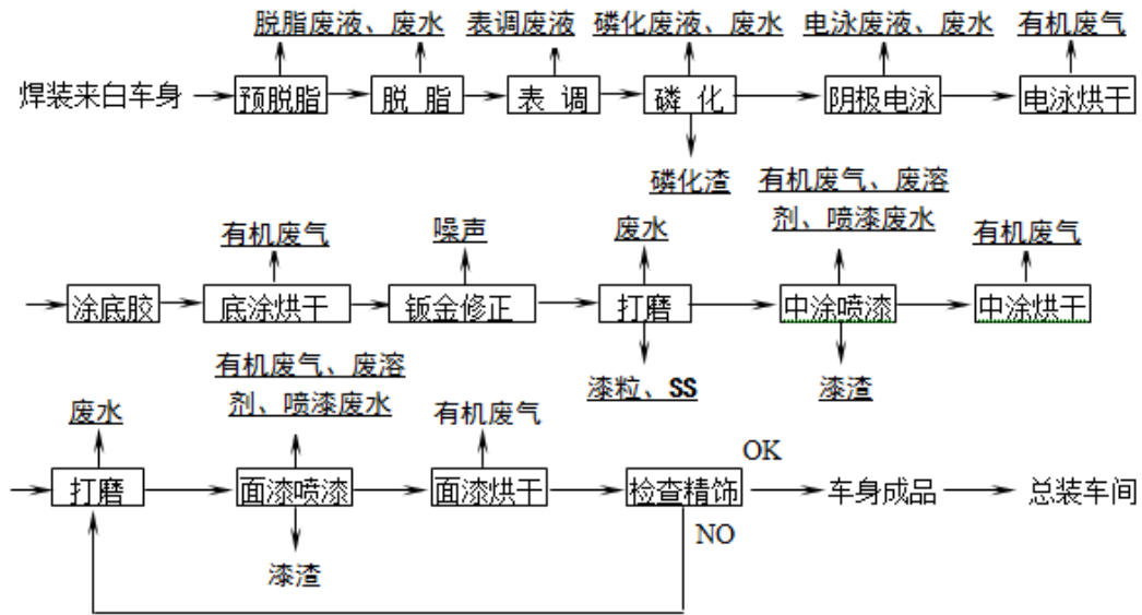
图 1-5 涂装生产工艺流程及产污节点图
