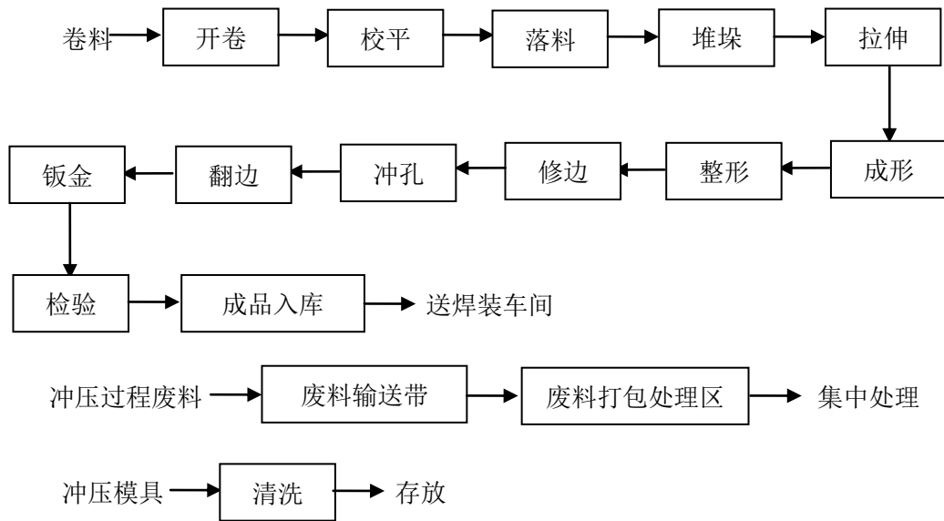
图 1-3 冲压生产工艺流程及产污节点图
