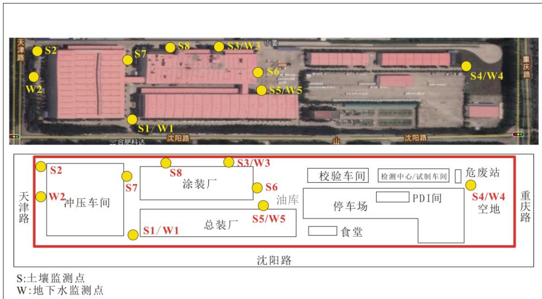
图 3-1 项目区采样点布置图
