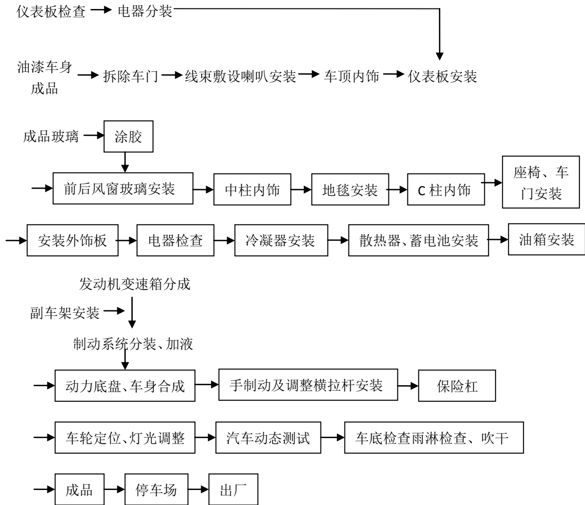
图 1-6 总装车间生产工艺流程图
