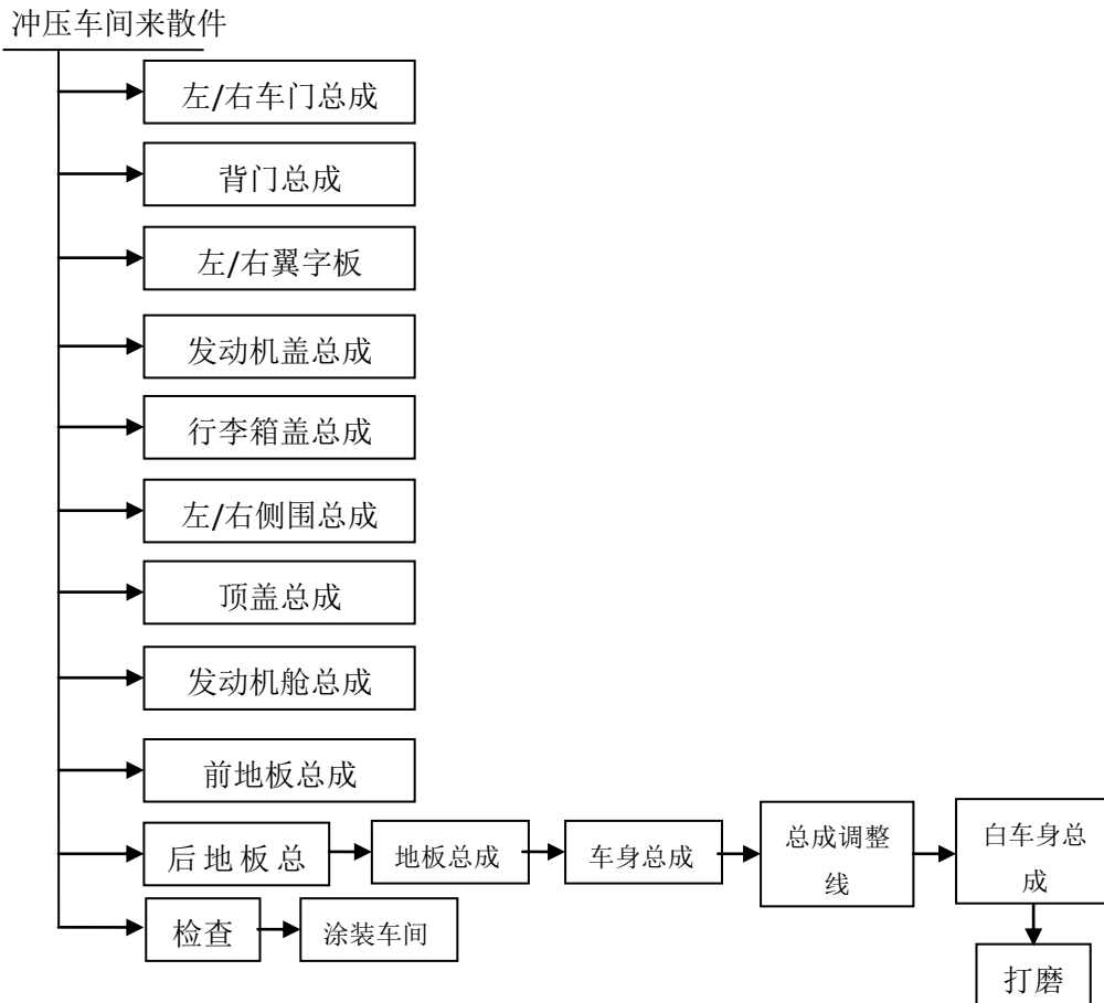
图 1-4 焊装生产工艺流程及产污节点图
